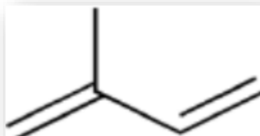
Figure 01 : Structure de l'unité isoprène ( Fillatre, 2011 )
